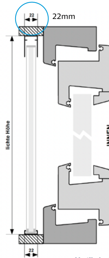
Vertikalschnitt
