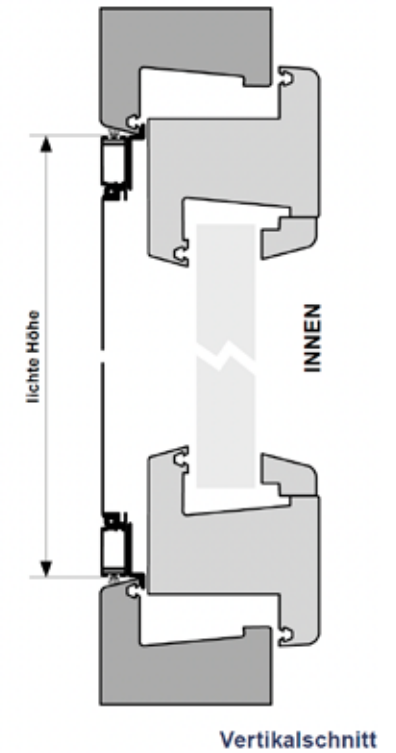
Spannrahmen 4013
