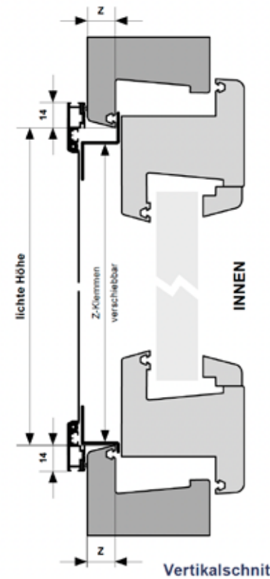
Spannrahmen 4010
